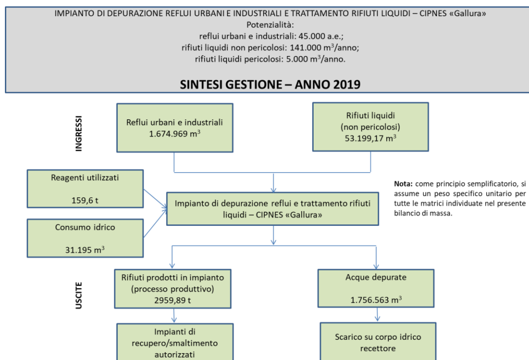
Figura 1: schema di flusso relativo all'esercizio dell'impianto consortile nell'anno 2019
